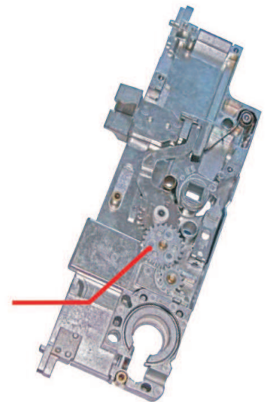
Mechanizm zamka na kołach zębatych
