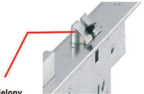
MACO-język dzielony Delikatny najazd w zaczep języka - gwarantuje pewne zamykanie drzwi
